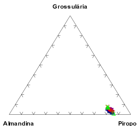
Figura 5.2.1. Composição das granadas dos granada lherzolitos.
