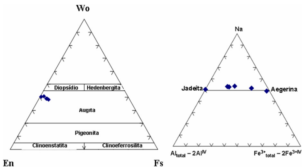
Figura 5.3.7: A) Classificação do clinopiroxênio do granada clinopiroxenito; B) Membros finais sódicos do clinopiroxênio do granada clinopiroxenito.
