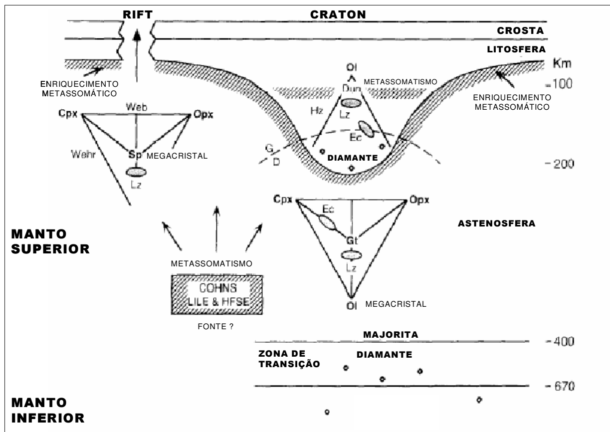
Figura 2.2. Seções esquemáticas do manto, mostrando os minerais maiores e os tipos de rochas esperadas no topo do manto inferior (670 – 2890 km), zona de transição (410 – 670 km) e manto superior (segmento abaixo da crosta: 0 - 10 km nos oceanos e 35 – 50 km em rifts e bordas de crátons e ~ 200 km nos centros dos crátons,. Kimberlitos e xenólitos associados são sub-cratônicos e os basaltos alcalinos ocorrem em rifts . Abreviações: EC (eclogito), LZ (lherzolito), HZ (harzburgito), DUN (dunito), WEB (websterito), WEHR (wehrlito), COHNS (carbono, oxigênio, hidrogênio, nitrogênio, enxofre), LILE (elementos litófilos), HFSE (High Field Strength Elements), GT (granada), CPX (clinopiroxênio), OPX (ortopiroxênio), SP (espinélio), OL (olivina), D (diamante), G (grafita). Modificado de Haggerty (1995).
