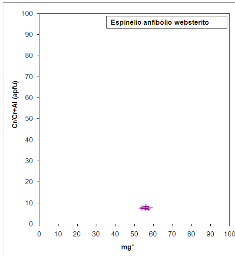
Figura 5.6.2. Correlação entre mg# e Cr/Cr + Al em espinélios do espinélio anfibólio websterito.
