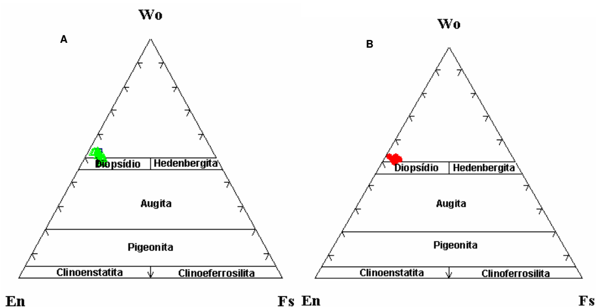
Figura 5.3.4. Classificação do clinopiroxênio do anfíbólio granada websterito (A) e espínélio anfibólio websterito (B).
