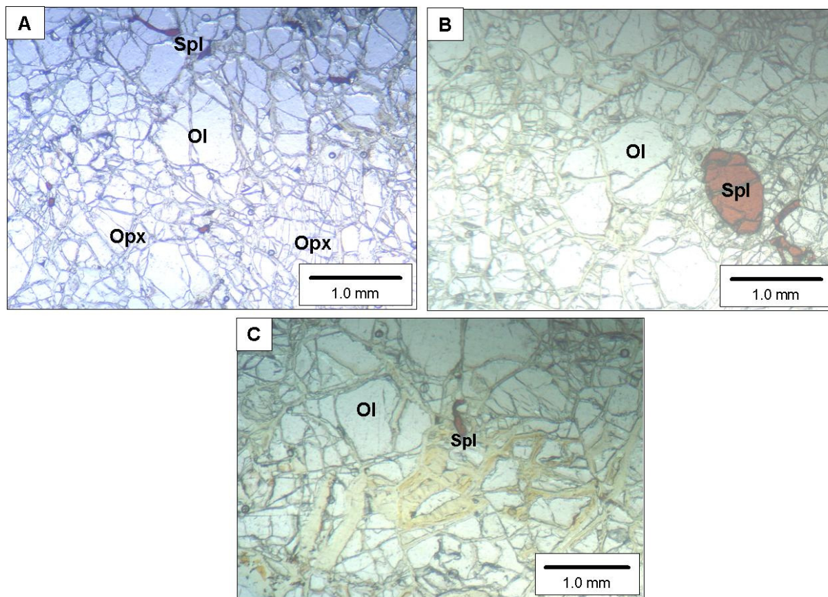
Figura 4.3. Fotomicrografias de espinélio harzburgitos: A) textura granoblástica formada por olivina e ortopiroxênio muito fraturados e espinélio disseminado; B) espinélio com forma arredondada e olivina fraturada; C) espinélio irregular. Nota-se um material fino entre os grãos, formado por serpentina, clorita e talco.
