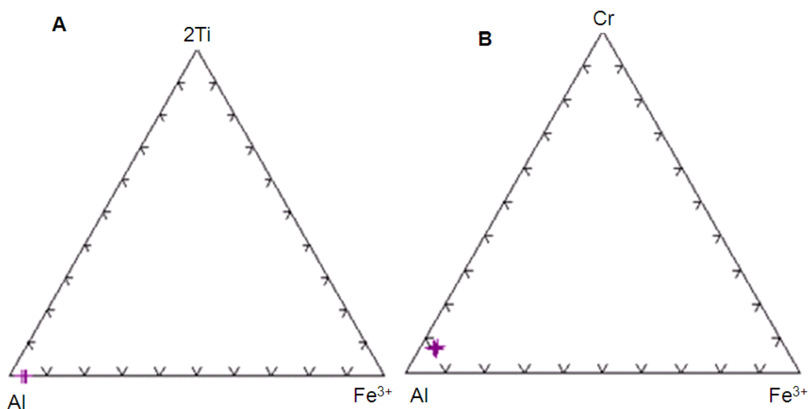
Figuras 5.6.3. Espinélio dos espinélio anfibólio websteritos: A) diagrama 2Ti - Al - Fe 3+ ; B) diagrama Cr - Al - Fe 3+ .
