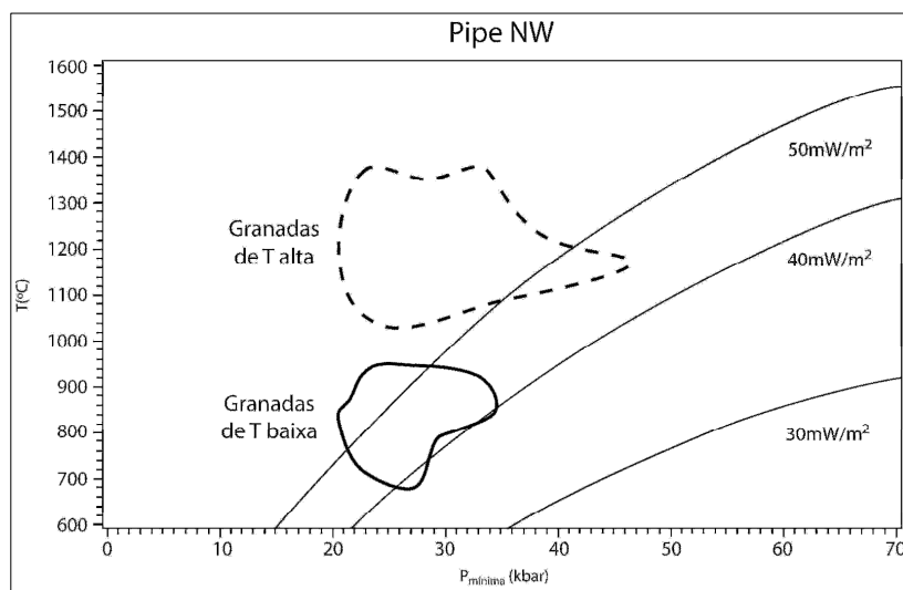
Figura 7.4. Campos P - T de granadas para o pipe NW do Canastra-01, obtidos por Winter (1997).
