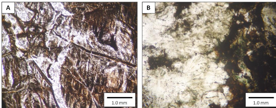
Figuras 4.8. Fotomicrografias de xenólitos alterados: A) amostra Can114; B) amostra Can134.
