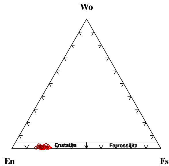
Figura 5.4.4. Classificação do ortopiroxênio do anfibólio granada websterito.
