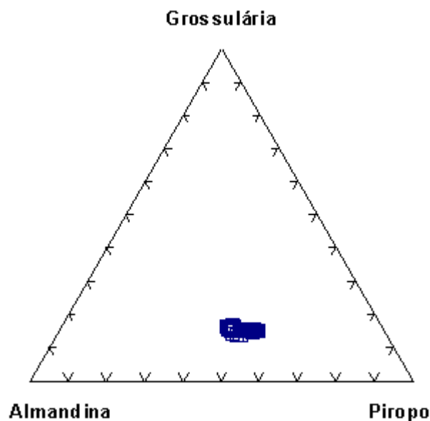
Figura 5.2.3. Composição das granadas do anfibólio granada websterito.
