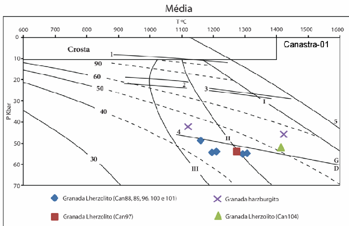
Figura 7.2. Diagrama contendo os valores das médias de P e T dos xenólitos do kimberlito Canastra-01. As curvas com valores de 30 a 90 representam as geotermas e seus respectivos valores de fluxo de calor em \text{mW/m}^2 ; as linhas pontilhadas indicam o aumento da transferência de calor por outros modos que não a condução (Pollack et al. , 1993). As linhas I, II e III são solidus para o manto e representam: I. ausência de voláteis; II. mistura de voláteis; III. presença de água (Pollack et al. , 1993). A área acima de 10 kbar corresponde à crosta. (Pollack et al. , 1993). As linhas 1, 2 e 3 correspondem a: 1- limite entre as fácies plagioclásio e espinélio; 2 e 3- limite da fácies espinélio e granada, as linhas paralelas em 2 e 3 representam “granada in ” (menor P ) e “espinélio out ” (maior P ); 5. solidus para o manto, segundo Hirschmann (2000). A linha G/D indica o limite grafita-diamante de Kennedy e Kennedy (1976).
