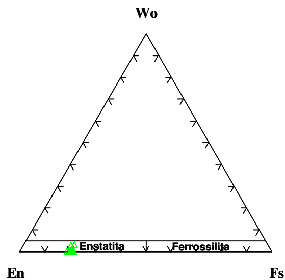
Figura 5.4.6. Classificação do ortopiroxênio do anfibólio websterito.
