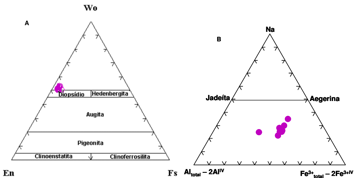
Figura 5.3.6: A) Classificação do clinopiroxênio do anfibólio websterito; B) Série dos membros finais dos clinopiroxênios do anfibólio websterito.
