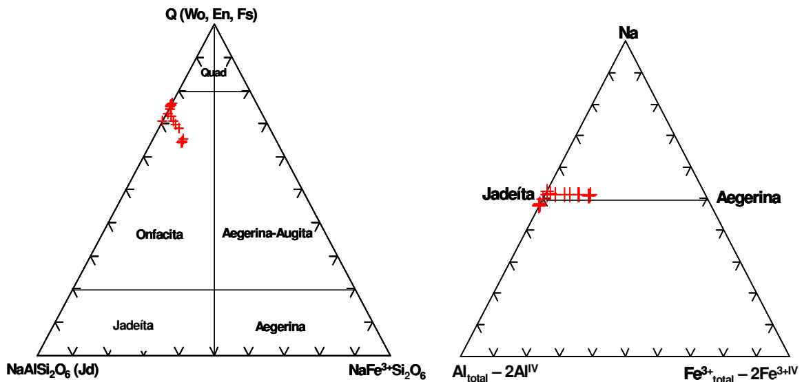
Figura 5.3.8: A) Classificação dos clinopiroxênios dos eclogitos; B) Membros finais sódicos do clinopiroxênio do eclogito.
