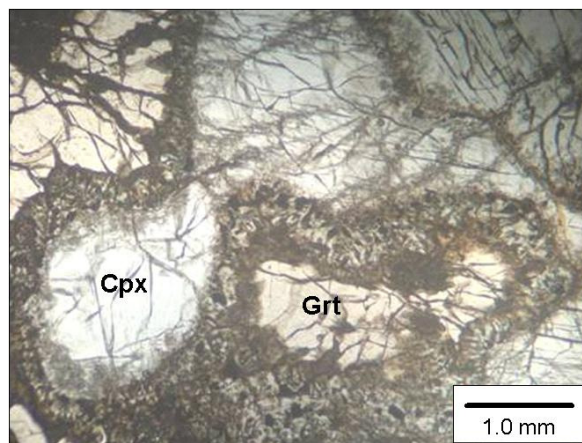
Figura 4.6. Fotomicrografia do granada clinopiroxenito, mostrando granulação grossa, constituída por granada e clinopiroxênio.
