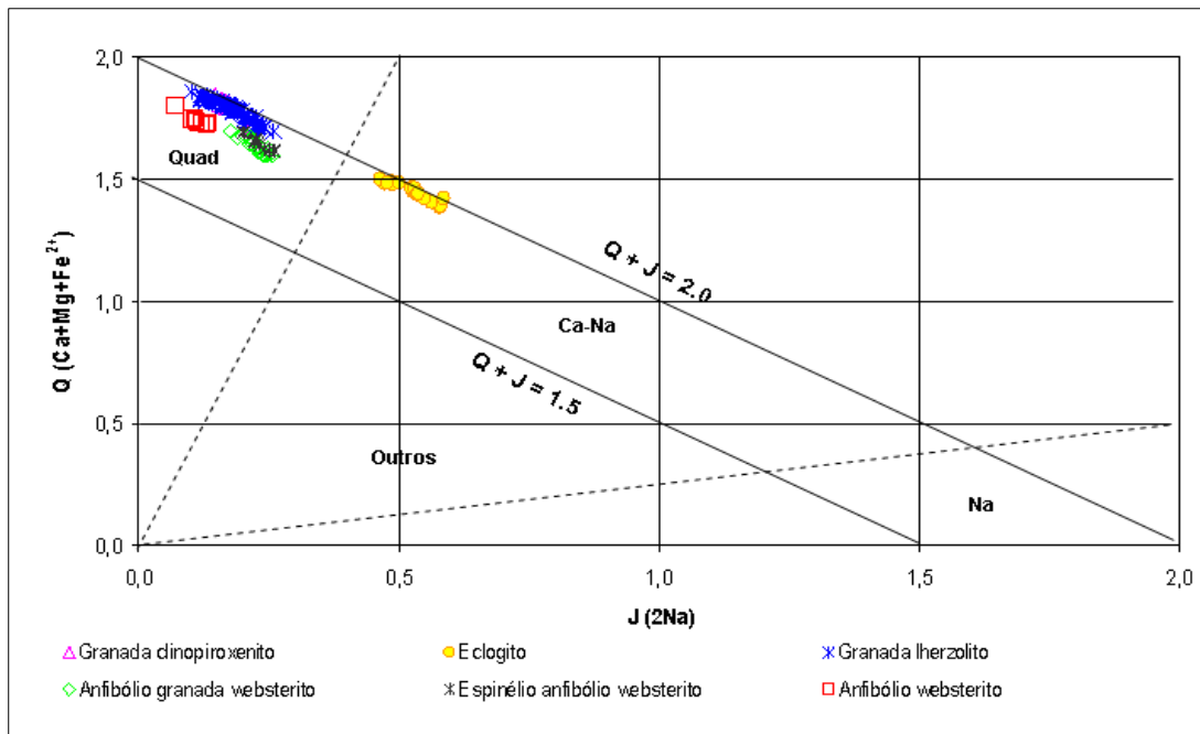
Figura 5.3.1. Diagrama Q-J para clinopiroxênios.
