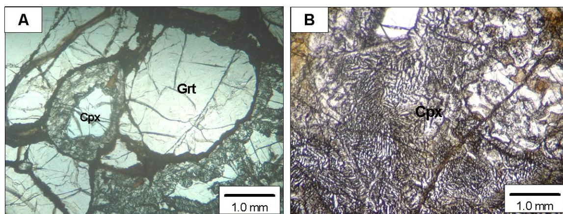
Figura 4.7. Fotomicrografias do eclogito: A) granada e clinopiroxênio arredondados. O contato entre os grãos se dá pela textura spongy do clinopiroxênio; B) clinopiroxênio alterado, exibindo textura spongy .
