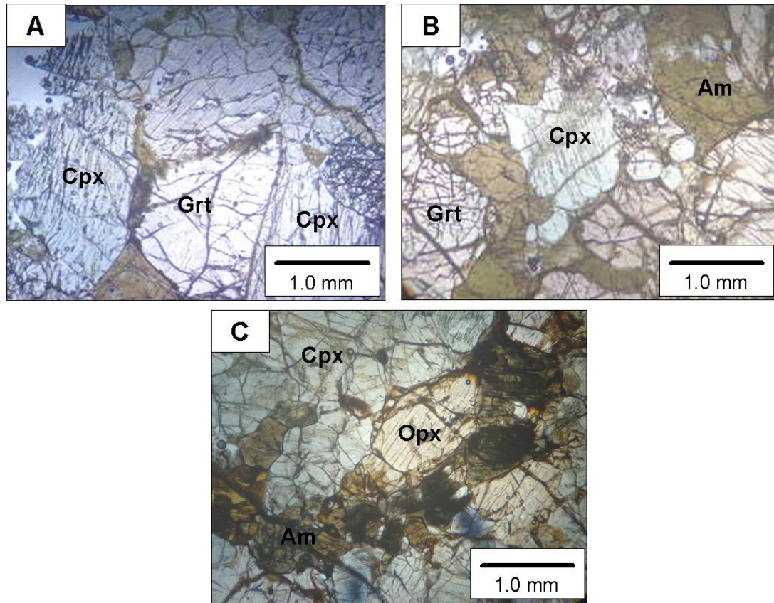
Figura 4.4. Fotomicrografias de anfibólio granada websterito: A) granada em contato com clinopiroxênio; B) clinopiroxênio e granada em contato com anfibólio; C) ortopiroxênio em contato com clinopiroxênio e anfibólio.
