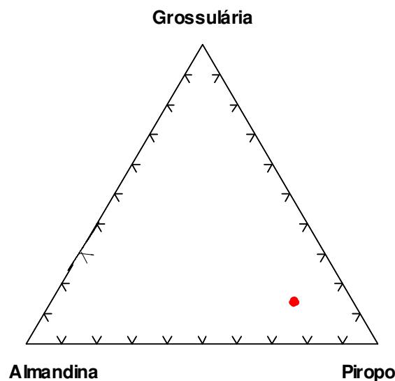
Figura 5.2.4. Composição da granada do granada clinopiroxenito.
