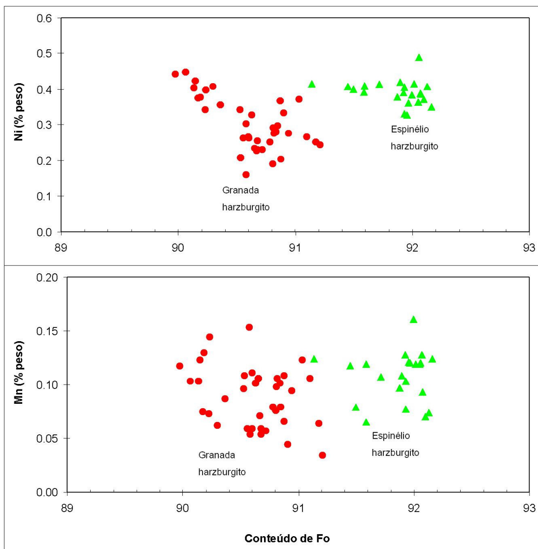
Figura 5.5.2. Diagrama forsterita versus Ni e Mn em granada e espinélio harzburgitos.
