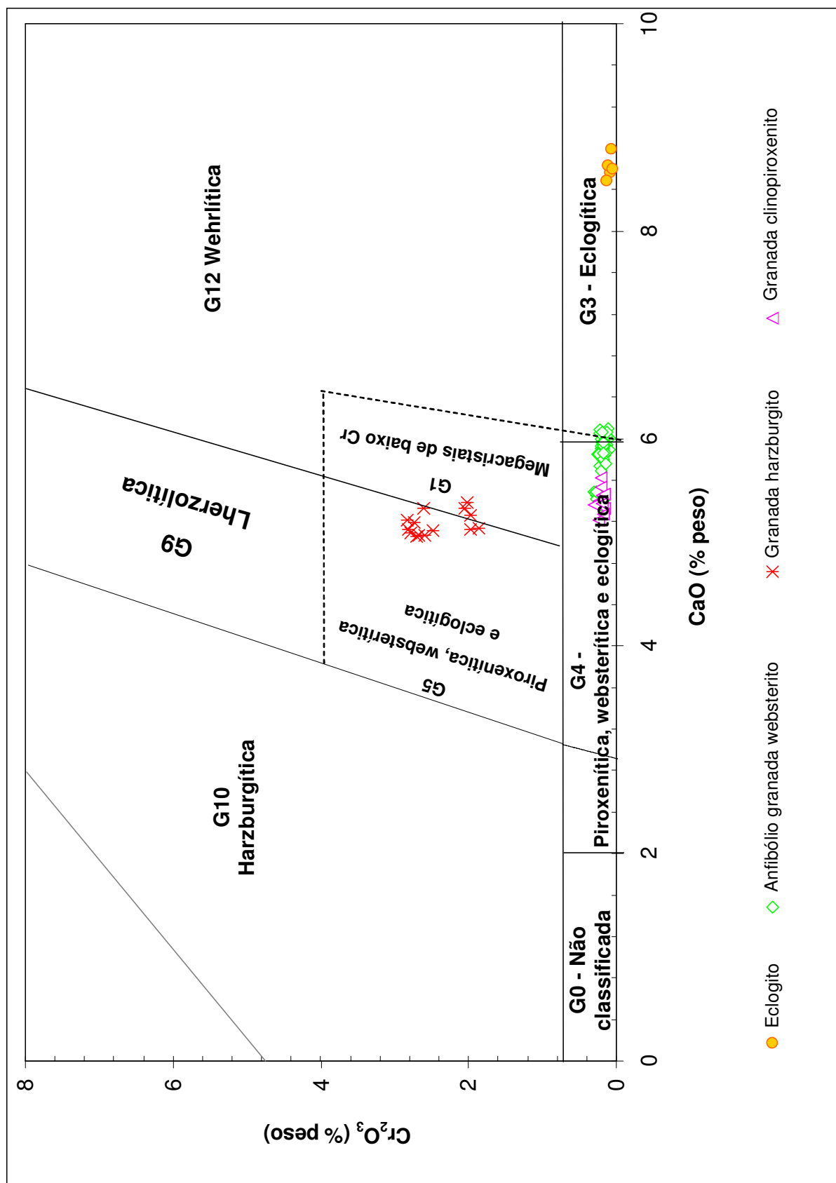
Figura 5.1. B. Classificação de granadas em diagrama \text{Cr}_2\text{O}_3 versus \text{CaO} das granadas dos xenólitos do Canastra-01, exceto as granadas dos granada lherzolitos, visando evidenciar que as granadas dos granada lherzolitos e granada harzburgitos estão sobrepostas.
