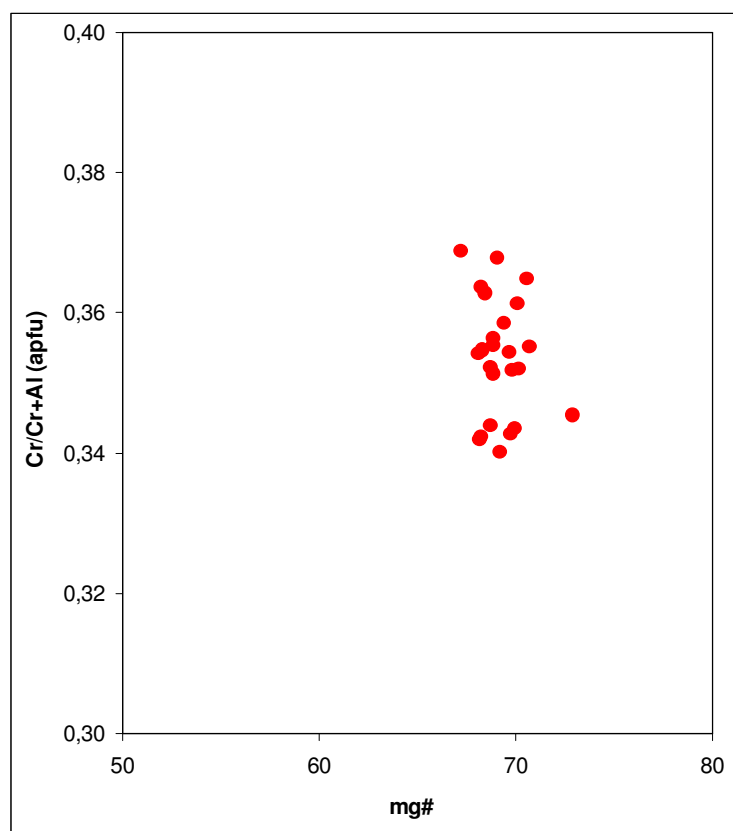
Figura 5.6.2. Correlação entre mg# versus Cr/(Cr+Al) para os espinélios do espinélio harzburgito.
