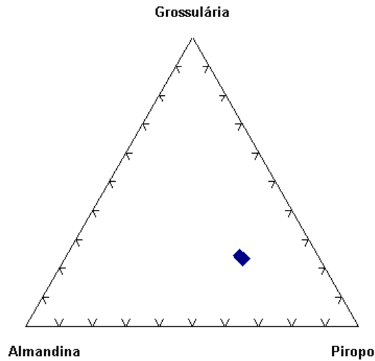
Figura 5.2.5. Composição da granada do eclogito.
