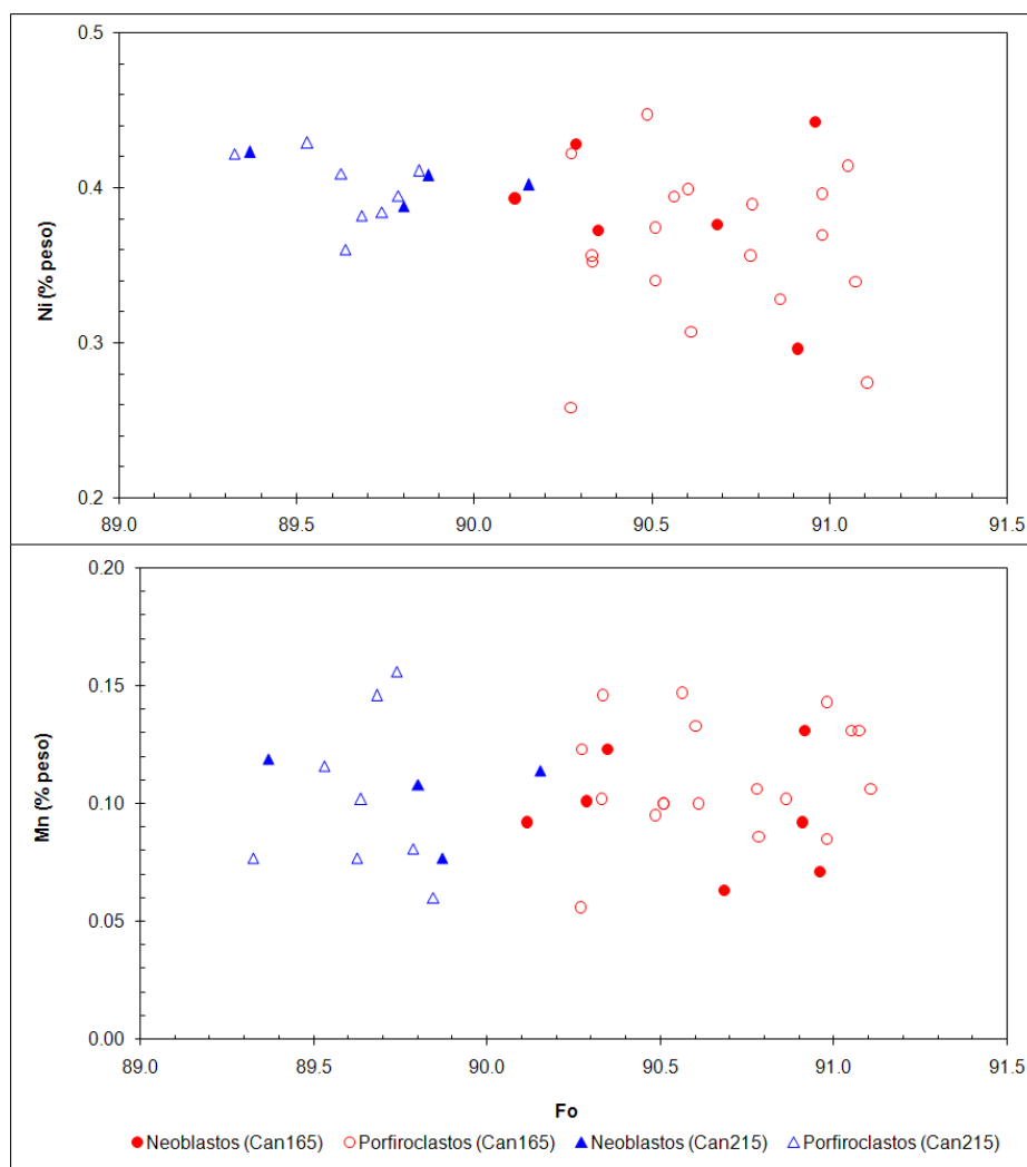
Figura 5.5.3. Diagrama Fo versus Ni e Mn das olivinas dos dunitos.
