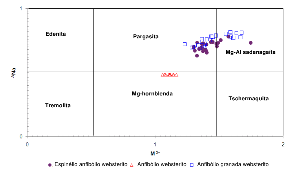
Figura 5.7.2. Classificação dos anfibólios das amostras de websterito. M^{3+} = Al + Fe^{3+} + Cr^{3+} + V^{3+} + Sc + 2*Ti^{4+} + 2*Zr no sítio M; ^ANa = conteúdo de Na no sítio A. Diagrama de Hawthorne e Oberti (2006).
