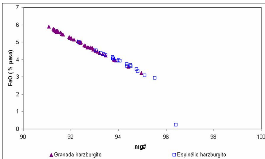
Figura 5.4.3. Correlação entre FeO versus mg# em ortopiroxênios dos harzburgitos.
