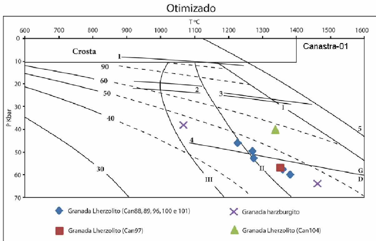
Figura 7.3. Diagrama contendo os valores otimizados de P e T dos xenólitos do kimberlito Canastra-01. As curvas com valores de 30 a 90 representam as geotermas e seus respectivos valores de fluxo de calor em \text{mW/m}^2 ; as linhas pontilhadas indicam o aumento da transferência de calor por outros modos que não a condução (Pollack et al. , 1993). As linhas I, II e III são solidus para o manto e representam: I. ausência de voláteis; II. mistura de voláteis; III. presença de água (Pollack et al. , 1993). A área acima de 10 kbar corresponde à crosta. (Pollack et al. , 1993). As linhas 1, 2 e 3 correspondem a: 1- limite entre as fácies plagioclásio e espinélio; 2 e 3- limite da fácies espinélio e granada, as linhas paralelas em 2 e 3 representam “granada in ” (menor P ) e “espinélio out ” (maior P ); 5. solidus para o manto, segundo Hirschmann (2000). A linha G/D indica o limite grafita-diamante de Kennedy e Kennedy (1976).
