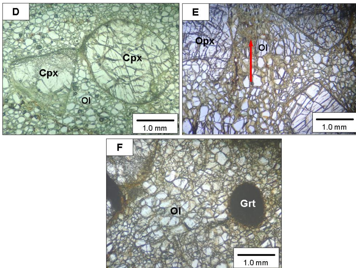
Figura 4.1. Fotomicrografias de granada Iherzolito: D) porfiroclastos de clinopiroxênio em matriz de mosaico de neoblastos de olivina. Nota-se estrutura de “quebra” que ocorre na borda do clinopiroxênio menor; E) grãos de olivina angulares e tabulares, mostrando uma orientação preferencial (como indica a seta). Nota-se material serpentínico entre os grãos; F) granada totalmente coberta por material quelifítico.
