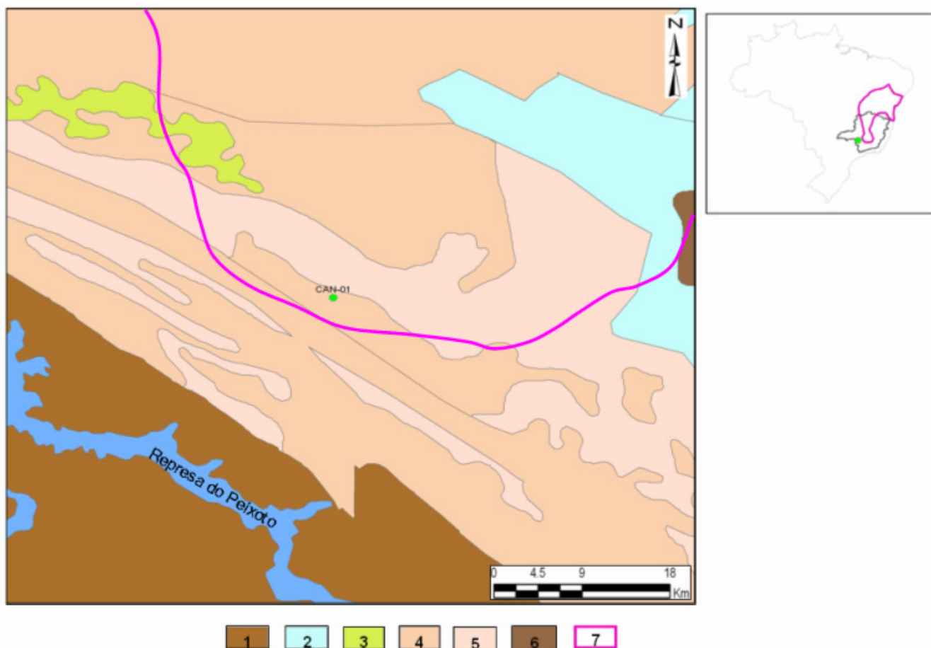
Figura 3.1. Mapa geológico da região do kimberlito Canastra 01: (1) Grupo Araxá; (2) Supergrupo São Francisco; (3) Grupo Bauru; (4) Grupo Canastra (quartzitos e filitos); (5) Grupo Canastra (domínio de xistos e filitos); (6) Grupo Bambuí – Fm. Jequitaí; (7) limite do Cráton São Francisco (compilado do banco de dados da De Beers Brasil Ltda.).
