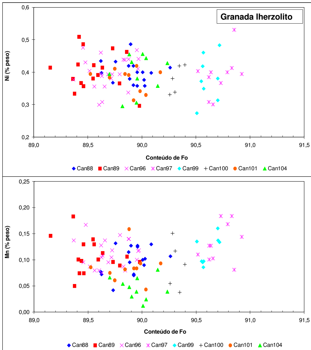
Figura 5.5.1. Diagramas forsterita versus Ni e Mn das amostras de granada lherzolito.
