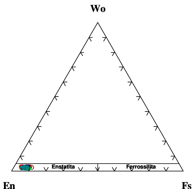
Figura 5.4.1. Classificação composicional do ortopiroxênio do granada lherzolito.
