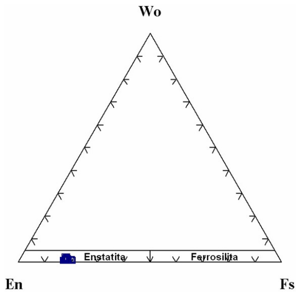
Figura 5.4.5. Classificação do ortopiroxênio do espinélio anfibólio websterito.
