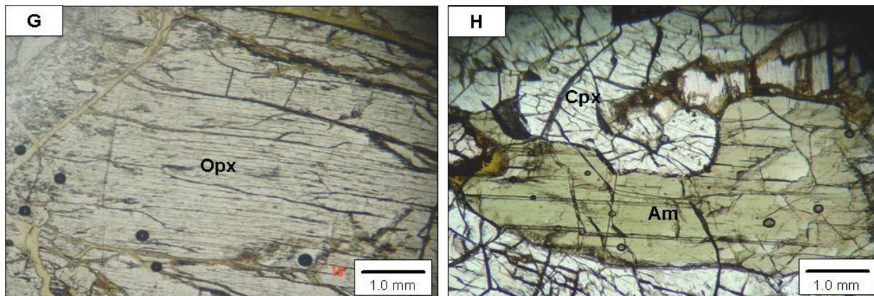
Figura 4.4. Fotomicrografias de anfibólio websterito: G) ortopiroxênio com fraturas preenchidas por material kimberlítico (?); H) clinopiroxênio e anfibólio exibindo textura granoblástica.
