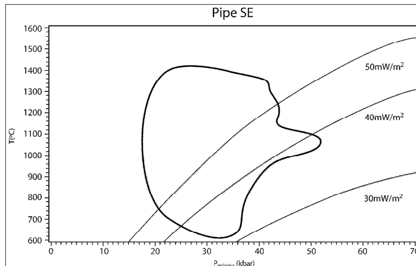
Figura 7.5. Campos P - T de granadas para o pipe SE do Canastra-01, obtidos por Winter (1997).
