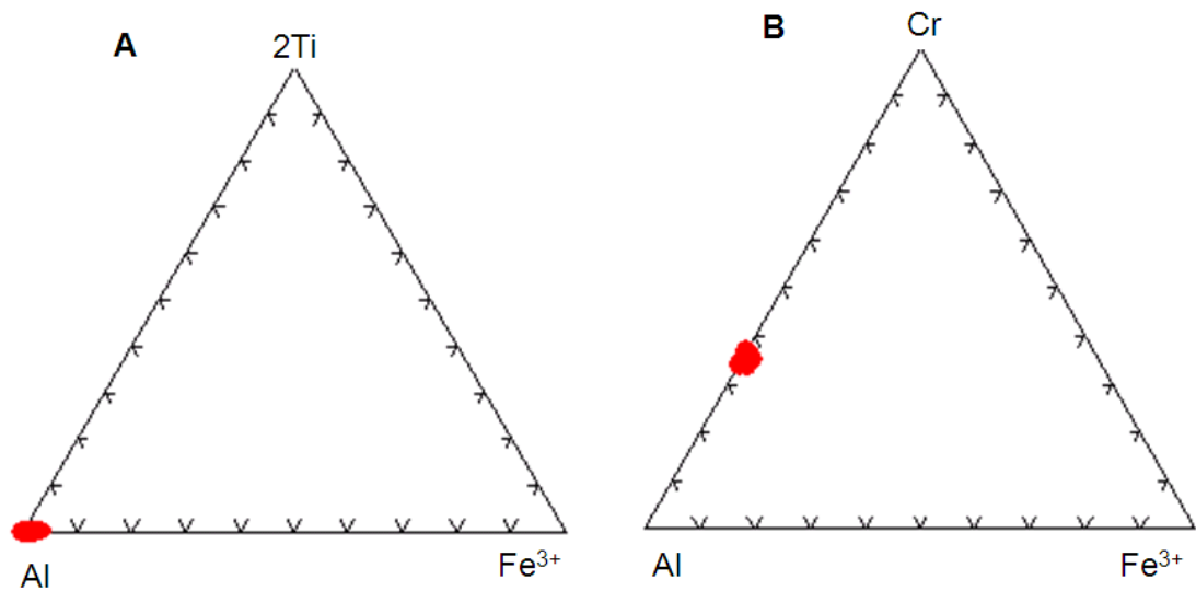
Figura 5.6.1. Espinélio do espinélio harzburgito: A) diagrama 2Ti - Al - Fe 3+ do espinélio dos espinélio harzburgito; B) diagrama Cr - Al - Fe 3+ do espinélio do espinélio harzburgito.
