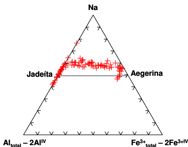
Figura 5.3.3. Membros finais dos clinopiroxênios dos granada lherzolitos.
