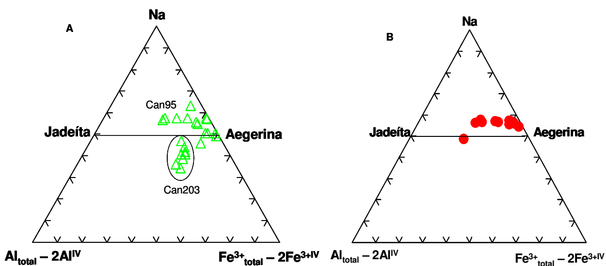
Figura 5.3.5. Série dos membros finais dos clinopiroxênios: A) anfíbólio granada websterito; B) espínélio anfibólio websterito.
