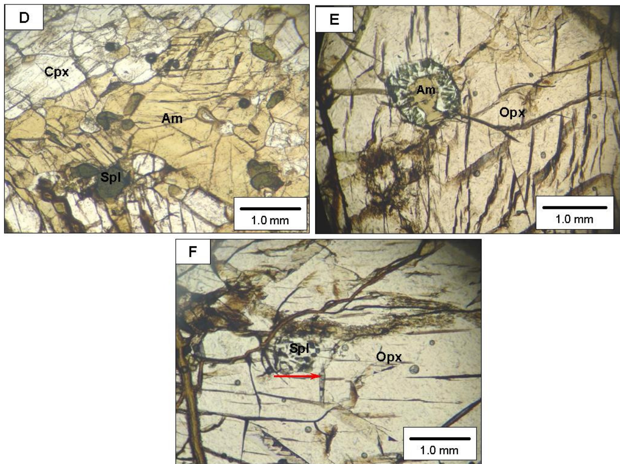
Figura 4.4. Fotomicrografias de espinélio anfibólio websterito: D) anfibólio e clinopiroxênio com grãos de espinélio verde disseminado; E) estrutura em corona no ortopiroxênio, constituída por espinélio de cor verde, clinopiroxênio incolor e anfibólio; F) espinélio com orientação preferencial (como indica a seta) dentro de ortopiroxênio.
