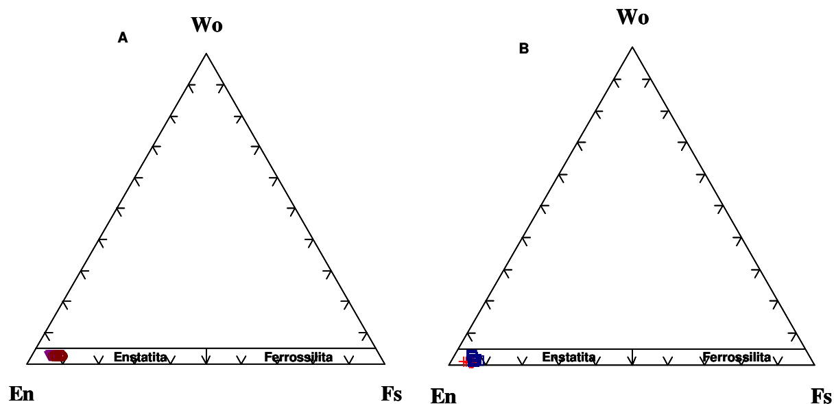
Figura 5.4.2. Classificação composicional dos ortopiroxênios: A) Granada harzburgito; B) Espinélio harzburgito.
