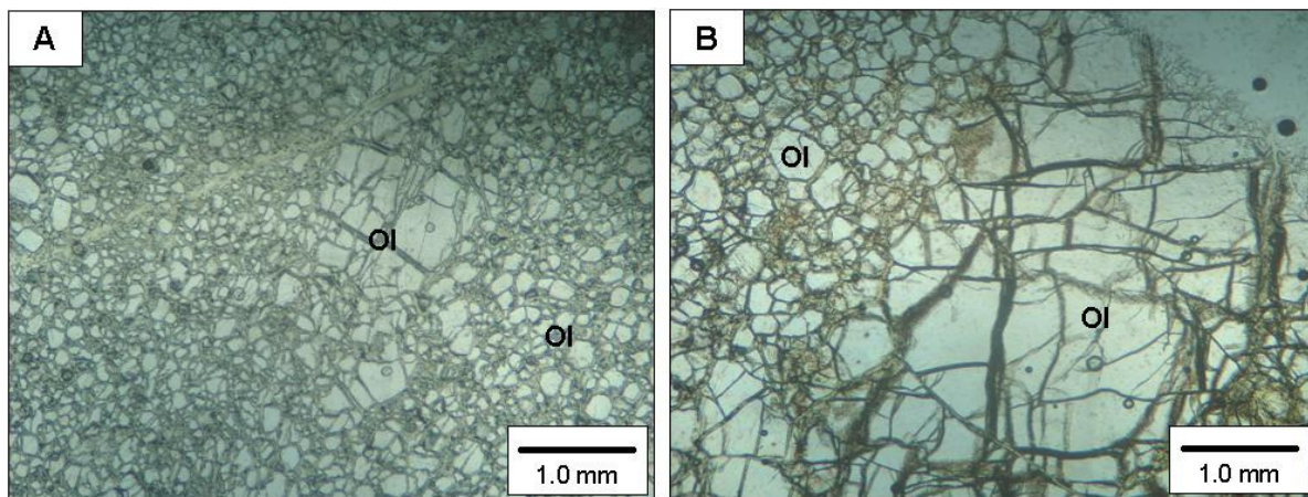
Figura 4.5. Fotomicrografias dos dunitos: amostras Can165 (A) e Can215 (B) - porfiroclasto de olivina em matriz equigranular de olivina.
