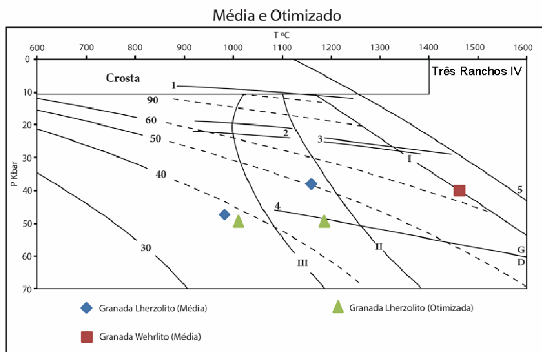
Figura 7.7. Diagrama contendo os valores das médias e otimizado de P e T dos xenólitos do kimberlito Três Ranchos IV. As curvas com valores de 30 a 90 representam as geotermas e seus respectivos valores de fluxo de calor em \text{mW/m}^2 ; as linhas pontilhadas indicam o aumento da transferência de calor por outros modos que não a condução (Pollack et al. , 1993). As linhas I, II e III são solidus para o manto e representam: I. ausência de voláteis; II. mistura de voláteis; III. presença de água (Pollack et al. , 1993). A área acima de 10 kbar corresponde à crosta. (Pollack et al. , 1993). As linhas 1, 2 e 3 correspondem a: 1- limite entre as fácies plagioclásio e espinélio; 2 e 3- limite da fácies espinélio e granada, as linhas paralelas em 2 e 3 representam “granada in ” (menor P ) e “espinélio out ” (maior P ); 5. solidus para o manto, segundo Hirschmann (2000). A linha G/D indica o limite grafita-diamante de Kennedy e Kennedy (1976).
