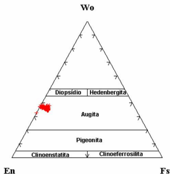
Figura 5.3.2. Classificação dos clinopiroxênios dos granada lherzolitos.
