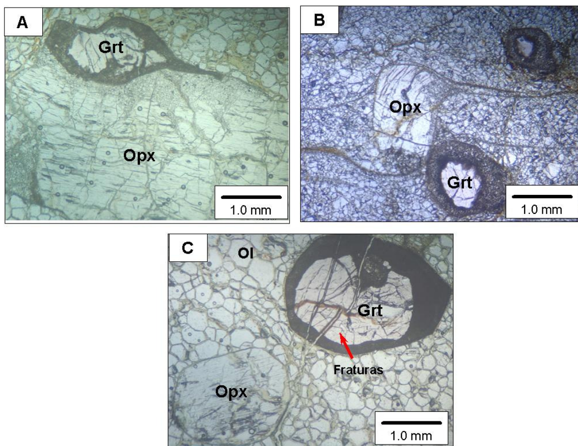
Figura 4.2. Fotomicrografias de granada harzburgitos: A) porfiroclasto de ortopiroxênio em contato sub-paralelo com granada; B) porfiroclasto de ortopiroxênio, que mostra franja de recrystalização; C) porfiroclastos de granada e ortopiroxênio arredondado, com matriz em mosaico de olivina. Fraturas tardias cortam a matriz e o porfiroclasto de granada (como indica a seta).
