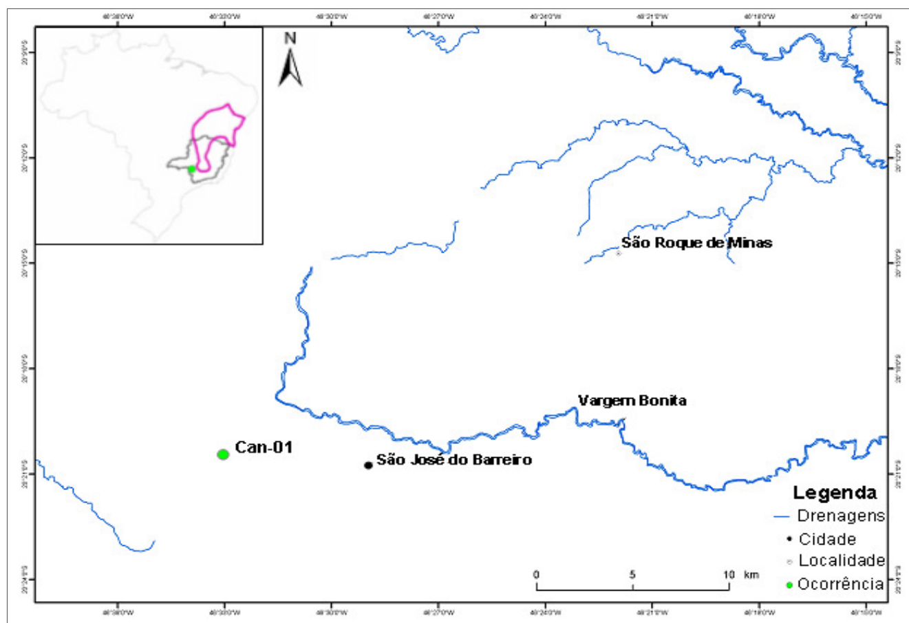
Figura 1. Localização do corpo Canastra – 01. Compilado do banco de dados da De Beers Brasil Ltda.
